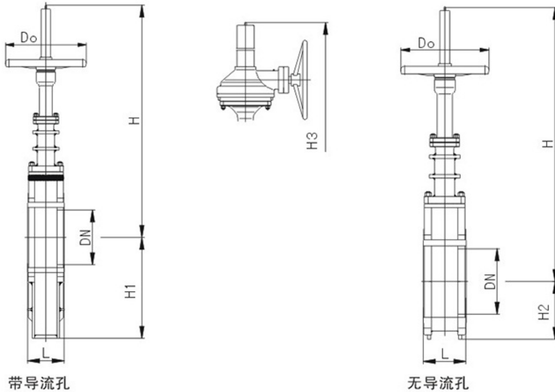
轻型平板闸阀主要外形尺寸及重量
