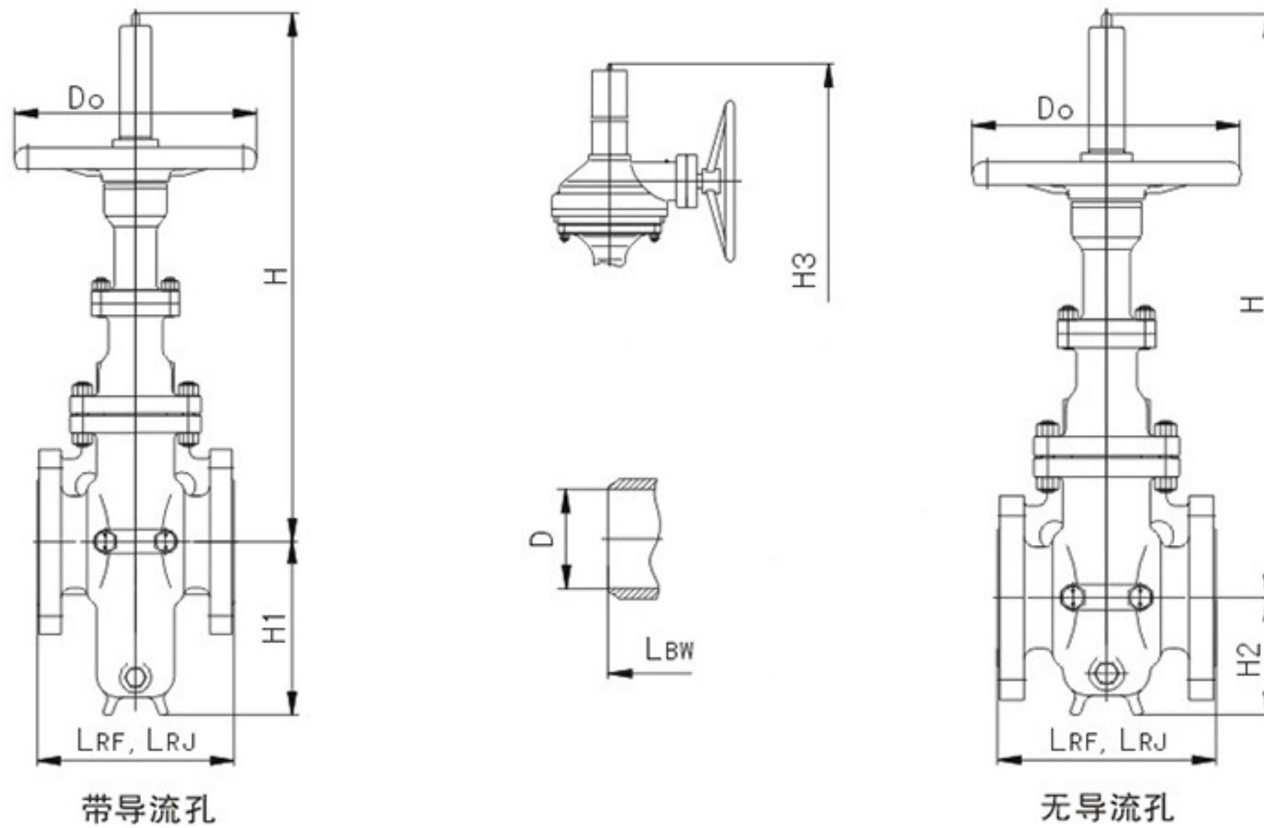
管线平板闸阀主要外形尺寸及重量
