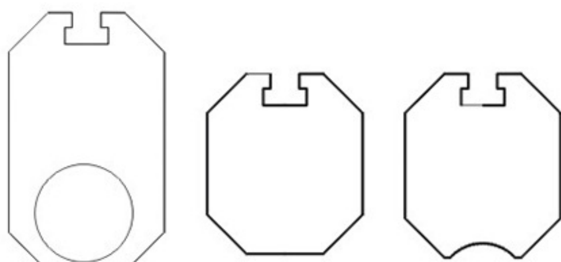
带导流孔型闸板 普通型闸板 调节型闸板
