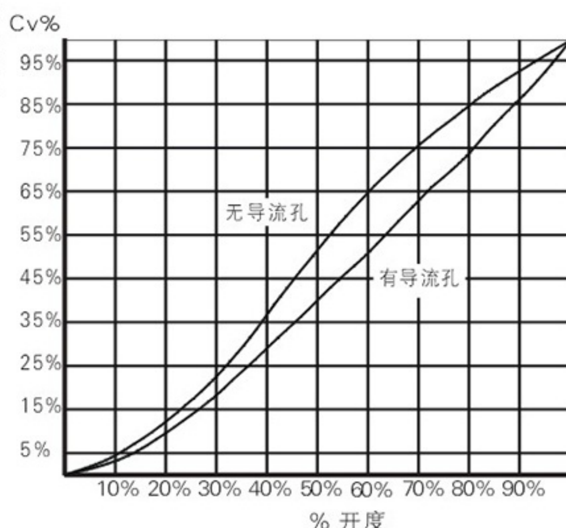
阀门开度-Cv特性曲线表
