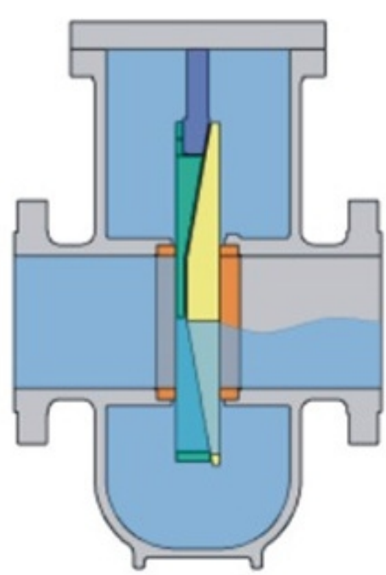
启闭运行状态
